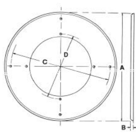
Afmetingen HAR-851 luidsprekerrooster: A=324mm; B=6mm; C=286mm; D=194mm
